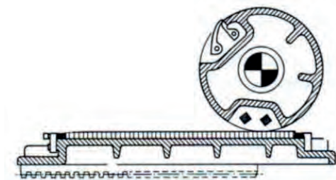
Afb. 2. Het drukfundament en de drukcilinder.
