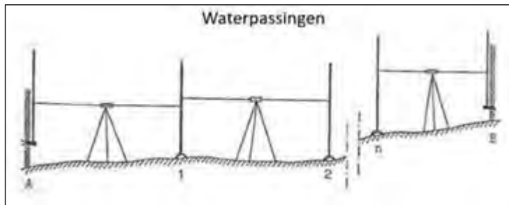
Afb. 5: Een principeschets van waterpassingen.
